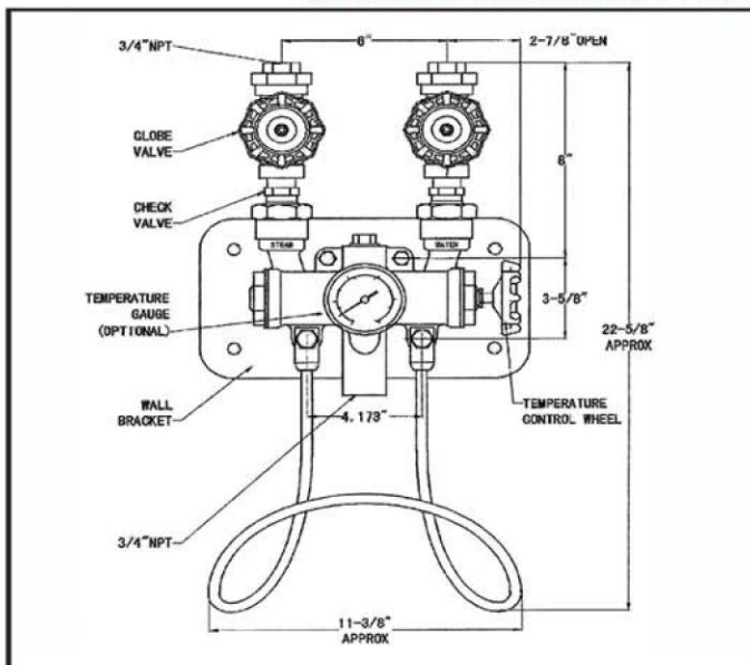
VISTA DELANTERA
